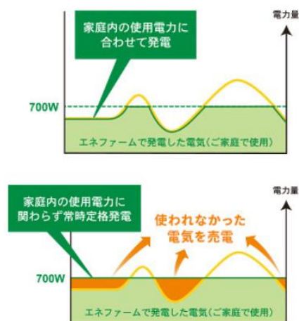
次世代エネファームの定格発電イメージ
